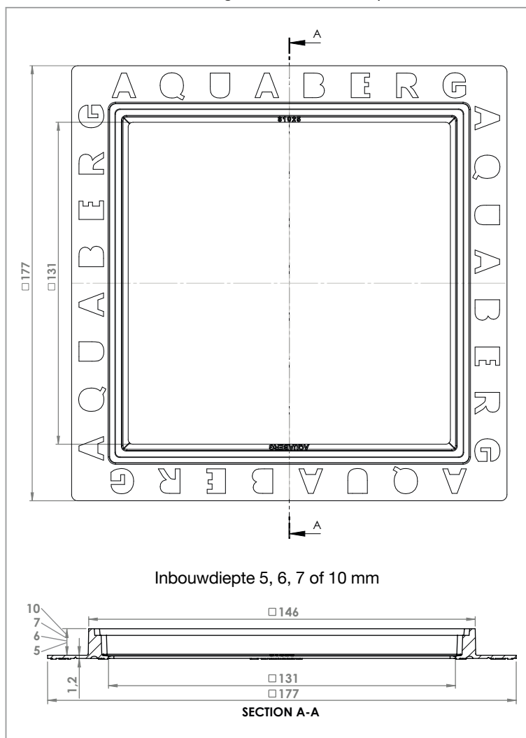
Maattekening kunststof renovatieput
